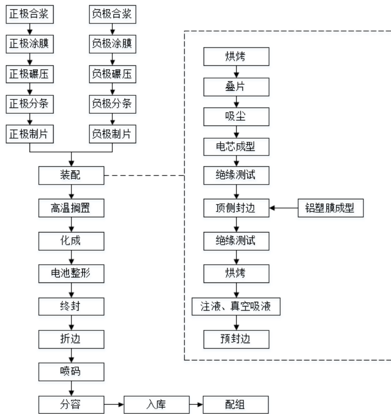
2、镍系电池生产工艺流程图
