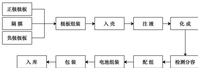
3、BMS 生产工艺流程图
